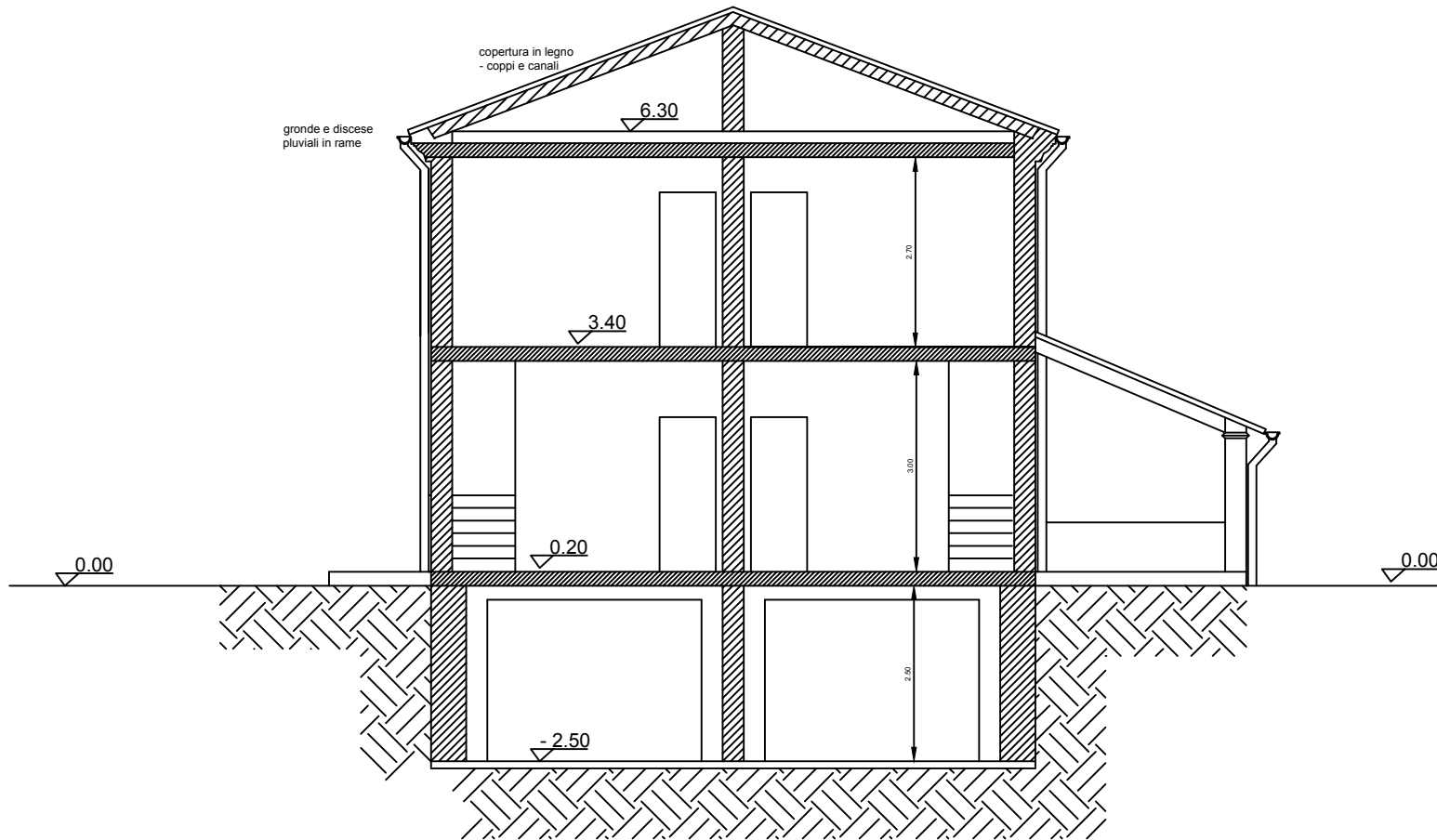
SEZIONE A-B 1:100
