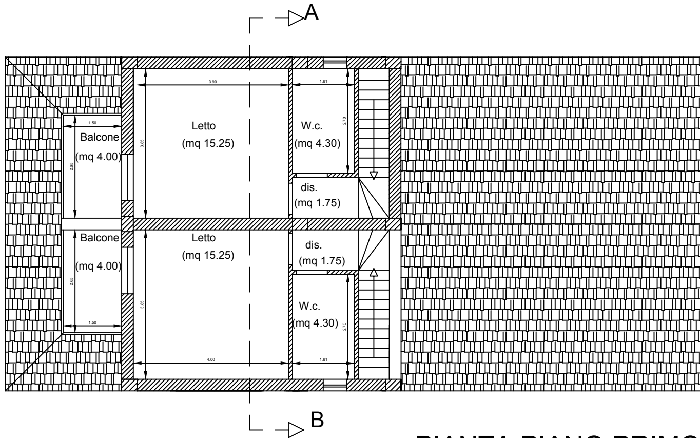
PIANTA PIANO PRIMO 1:100
